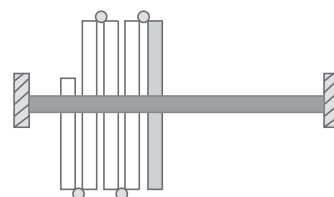
Configuración 5 hojas: Kit 2 hojas + 3 Kit+1 hoja
