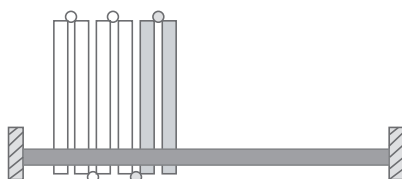
Configuración 6 hojas Kit 2 hojas + 2 Kit +2 hojas + 3 Guías Tauro
