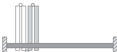
Configuración 4 hojas: Kit 2 hojas + Kit+2 hojas + 2 Guías Tauro
